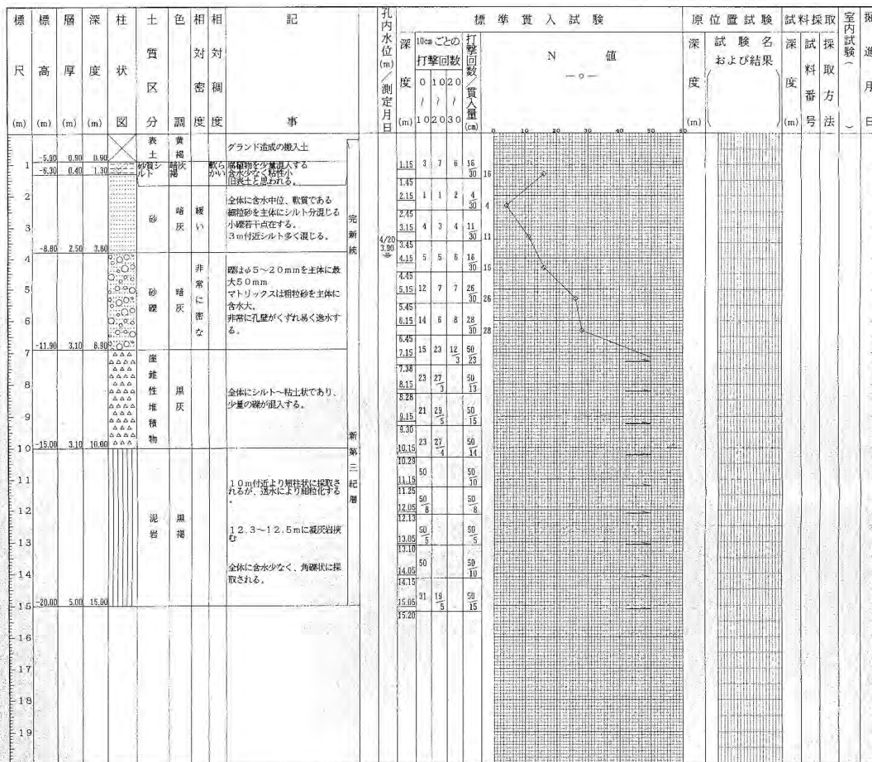
図 2.3.7(2) ボーリング柱状図 (No. 2)
