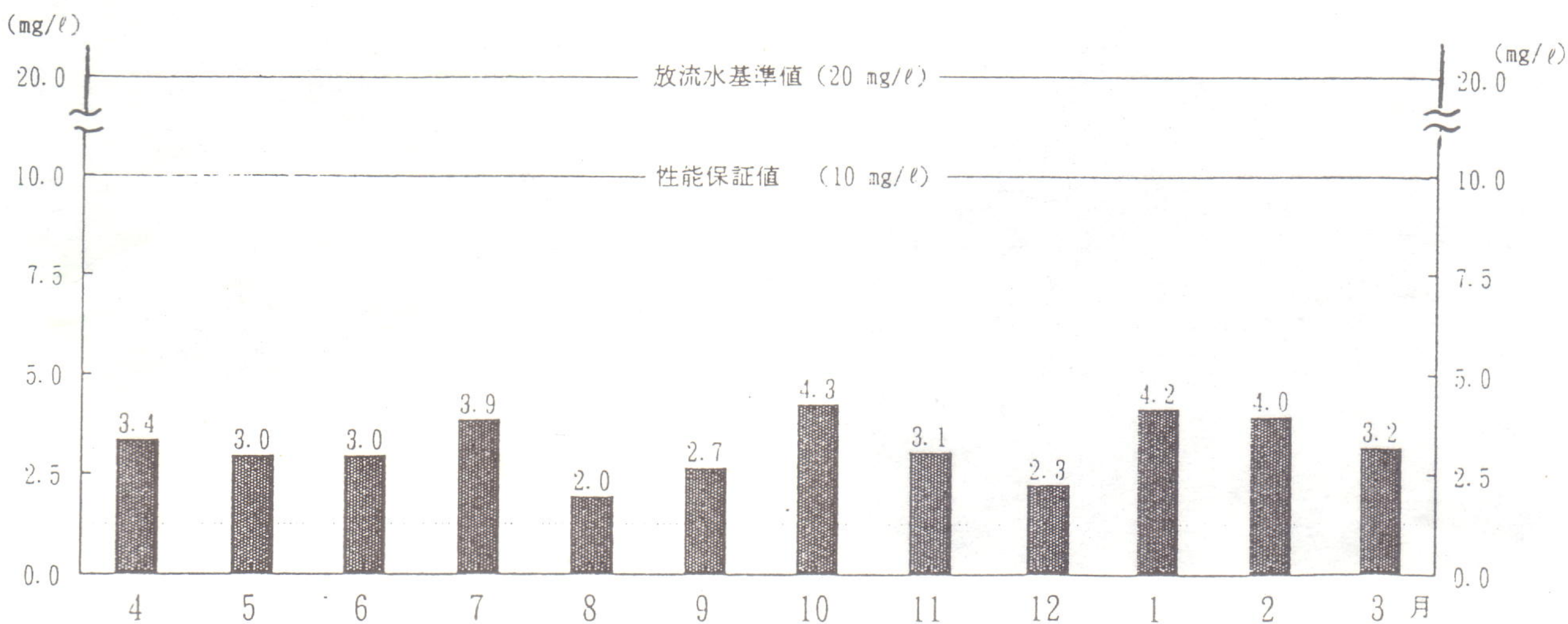
放流水のBOD実績値 (5年度)
